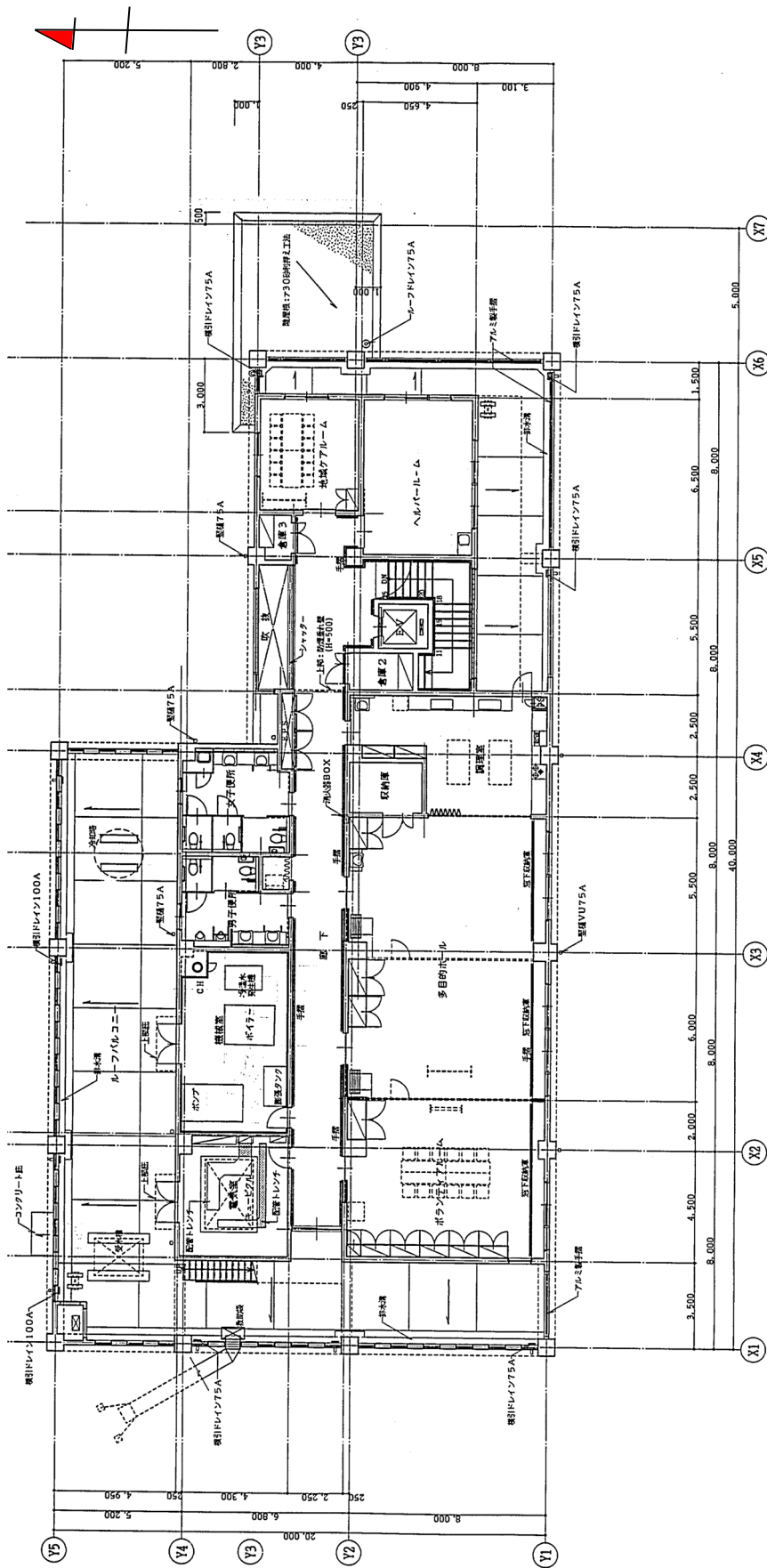
2階平面図
