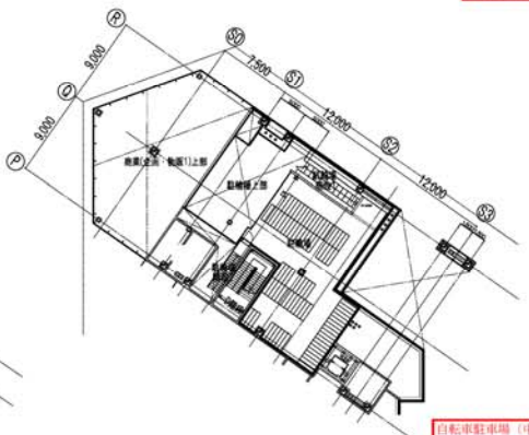
1階平面図 (FL+3,000)
