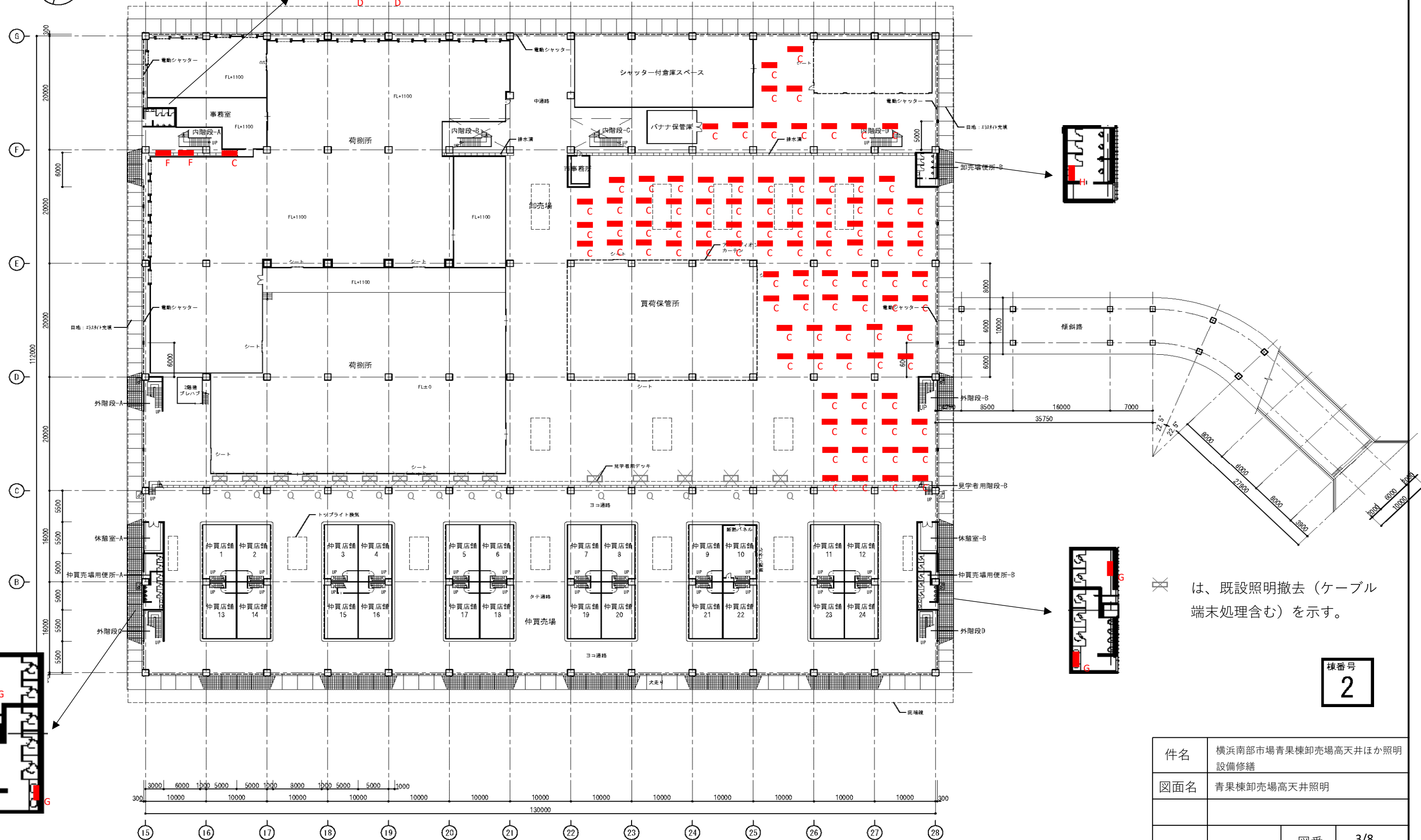
1階平面図
