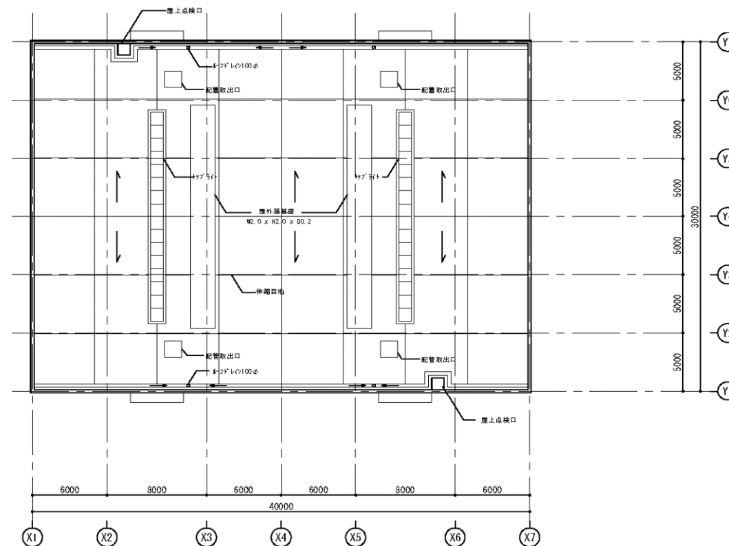
屋根伏図
