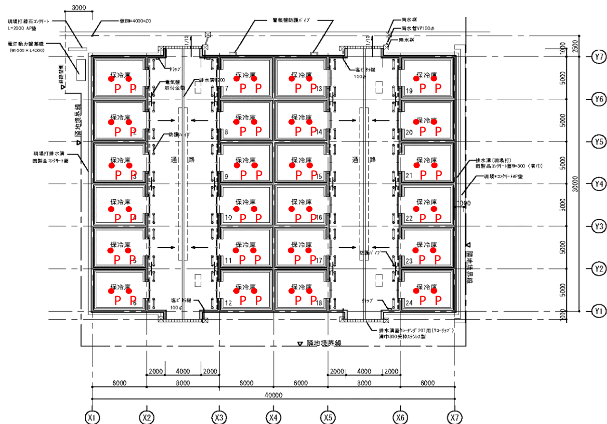
1階平面図
