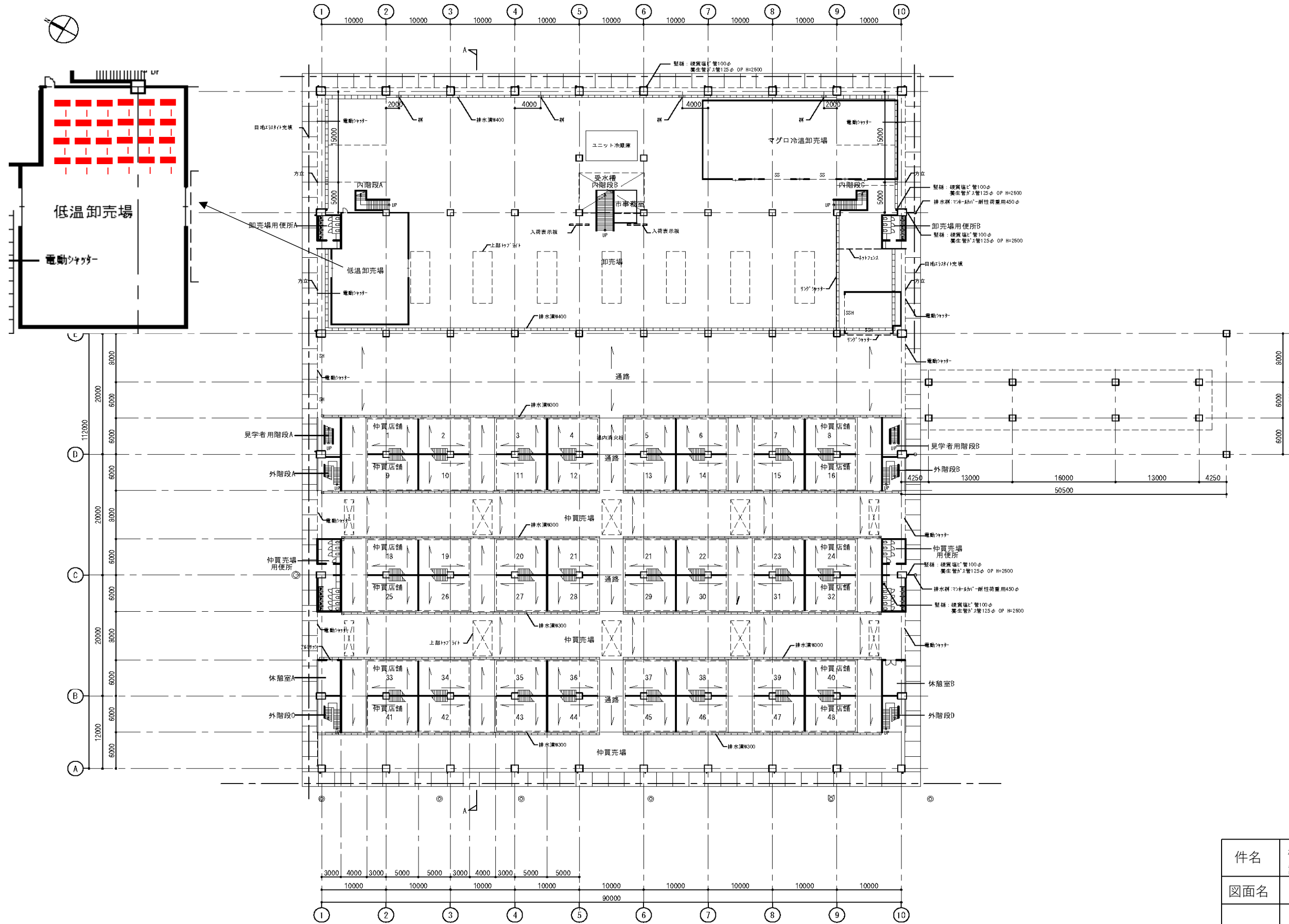
1階平面図
