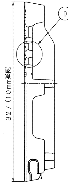
B-B断面図
