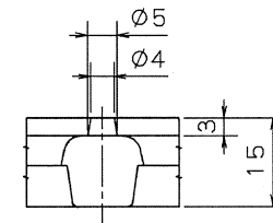
D部詳細図
