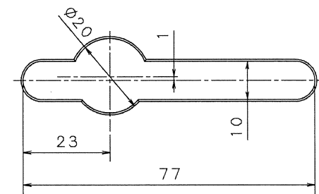
C部詳細図(手鍵穴)
