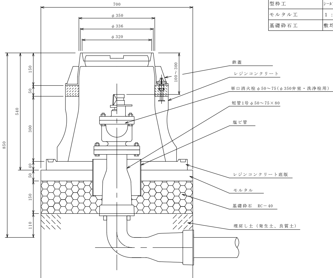
断面図
