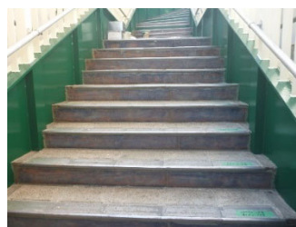
計画的な修繕の例(令和4年11月完成 南区 通町歩道橋)
