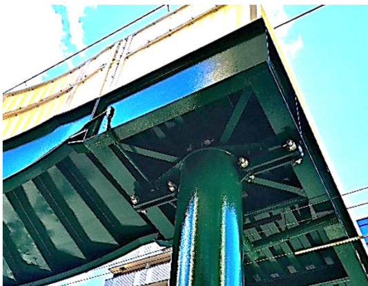
通町歩道橋(南区):落橋防止装置 令和4年11月完成
