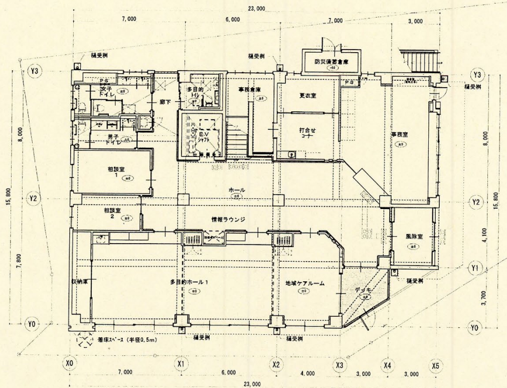
1階平面図
