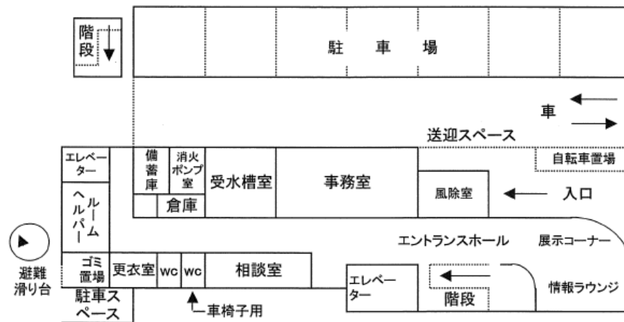
1階平面図
