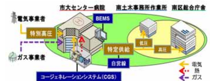
南区庁舎及び市大センター病院間のエネルギー連携
