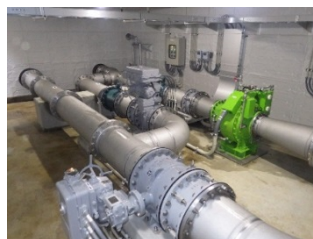
恩田配水池 小水力発電設備
